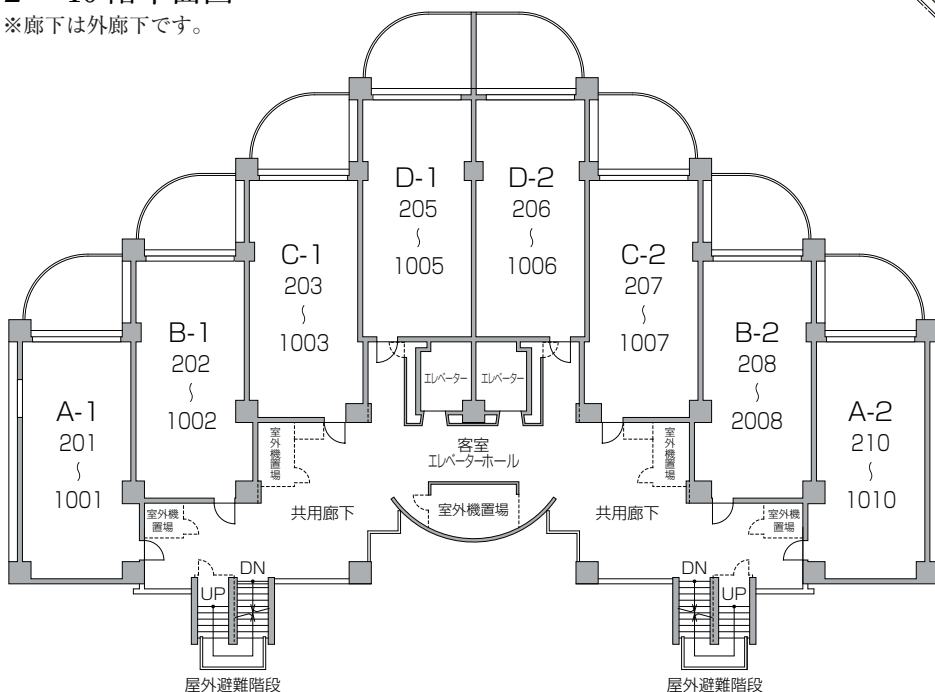
■ 2～10階平面図
